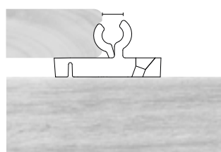
Verbinder-Vorspannung
