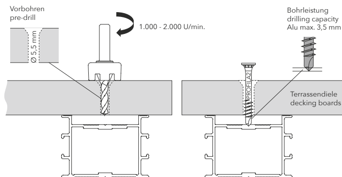
PROFILA2 Terrassendielen auf Aluminiumunterkonstruktion decking boards to aluminium substructures
