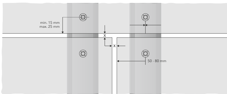
PROFILA1 Holzunterkonstruktion auf Stahlprofile | STEEL tube with wooden substructure
