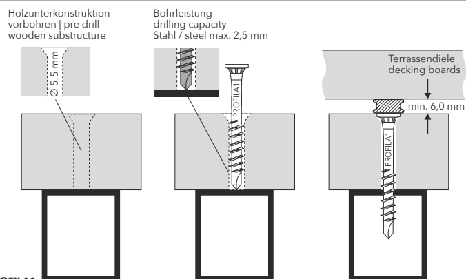
PROFILA1 Holzunterkonstruktion auf Stahlprofile | STEEL tube with wooden substructure
