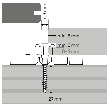
Groove-Profile
