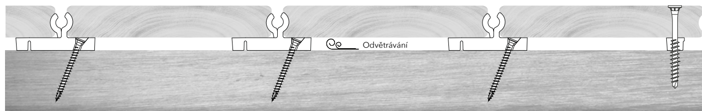
Zčásti viditelné šroubové spojení startovacího a koncového prkna
