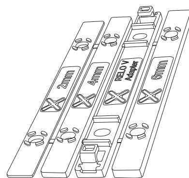
RELO VU Výškově nastavitelná sada
