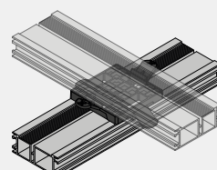
s RELO T56 stavební výška 60 mm*
