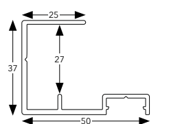
Sloupkový přípojovací profil PA 24 - 27 mm
